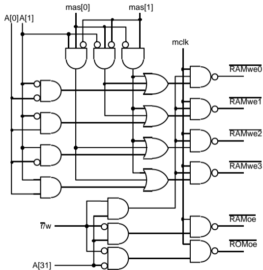
Adresdecoder Hardware
