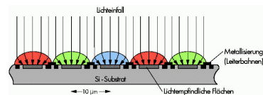
Linsensystem zur Kompensation der reduzierten Sensorfläche
